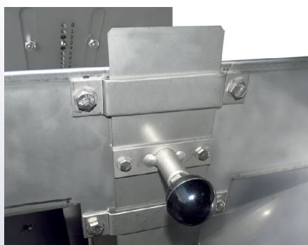
Alavanca de regulagem para vazão de ração com escala indicativa.
