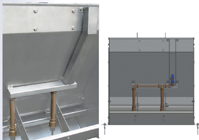
Tubo para entrada de água. Opção em aço inox ou PVC
